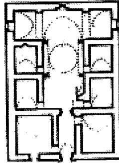
(تخطيط ١٧) : خانقاة بوياليكوى فى آفيون بأسيا الصغرى (الأناضول) من القرن ١٣/هـم (إيوان موسع بسدلتين ويسقف الصدر قبة) عن: (Akurgal (E.) : L'Art En Turquie , France 1981, Fig 30 . b -)
